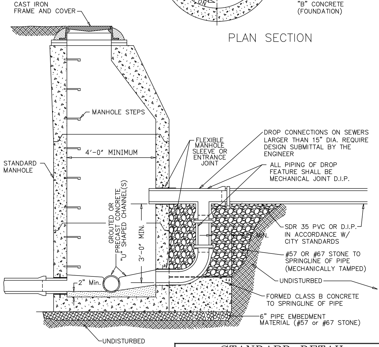
SECTION A-A
